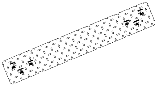
Cardboard template Plantilla
